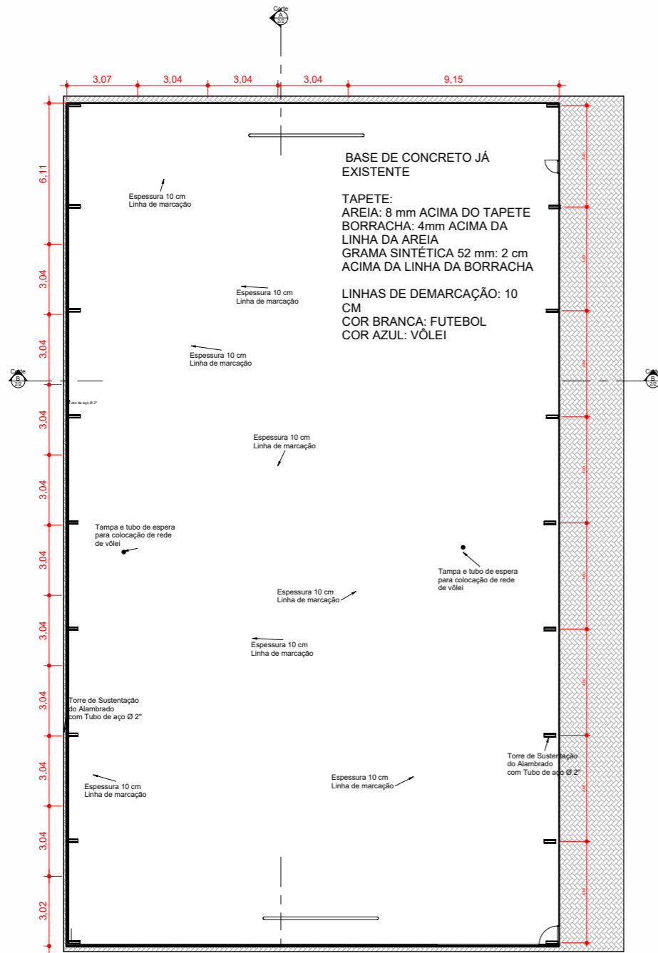
1 Planta Baixa 1:75
