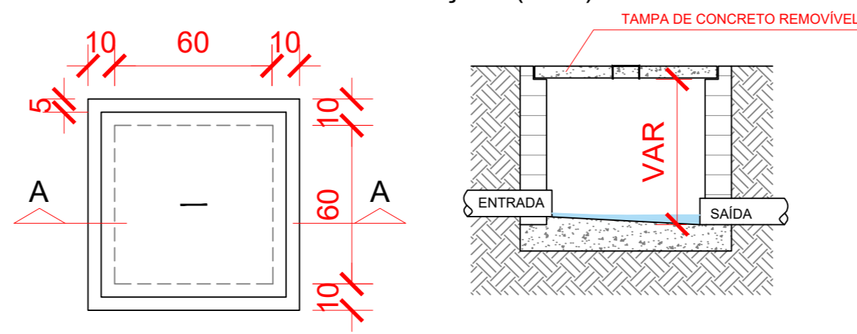
PLANTA BAIXA ESCALA 1:20
