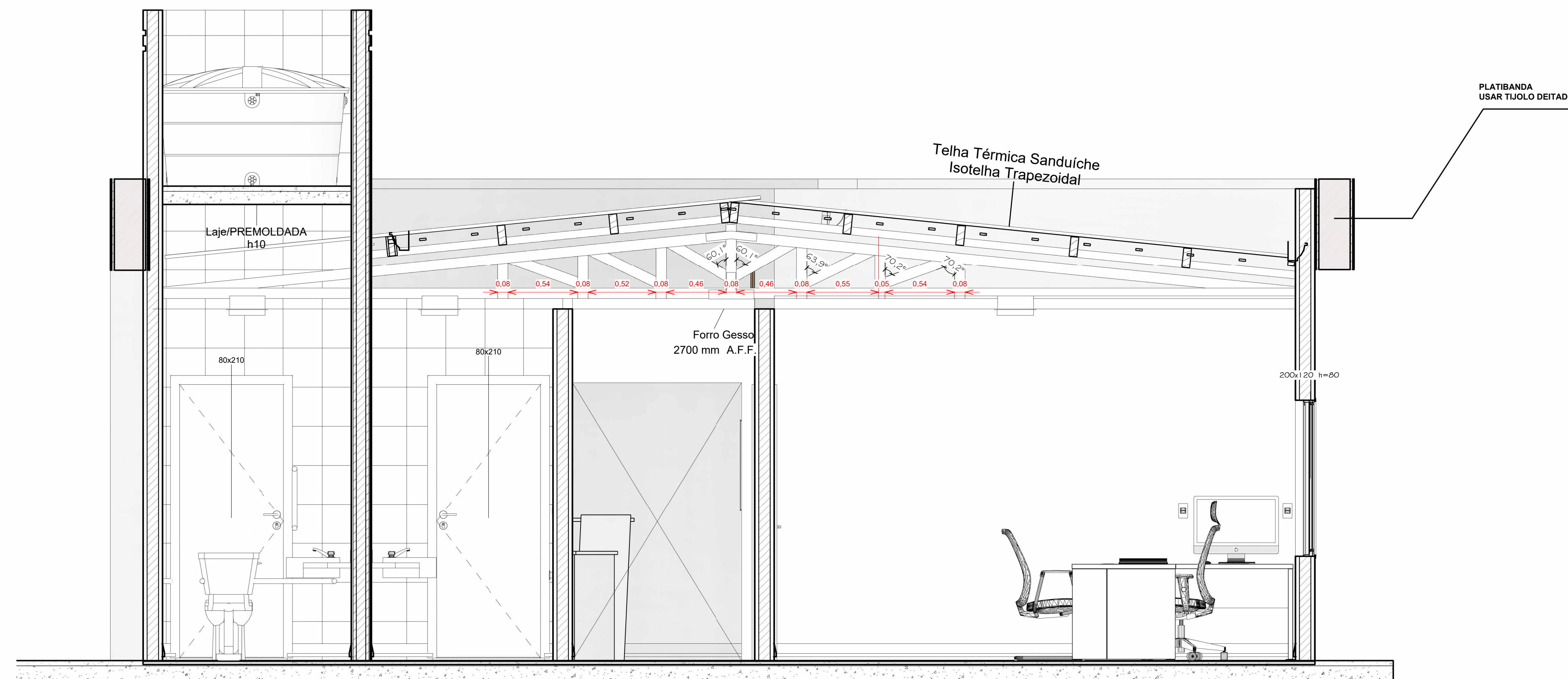
1 CORTE 02 1 : 20
