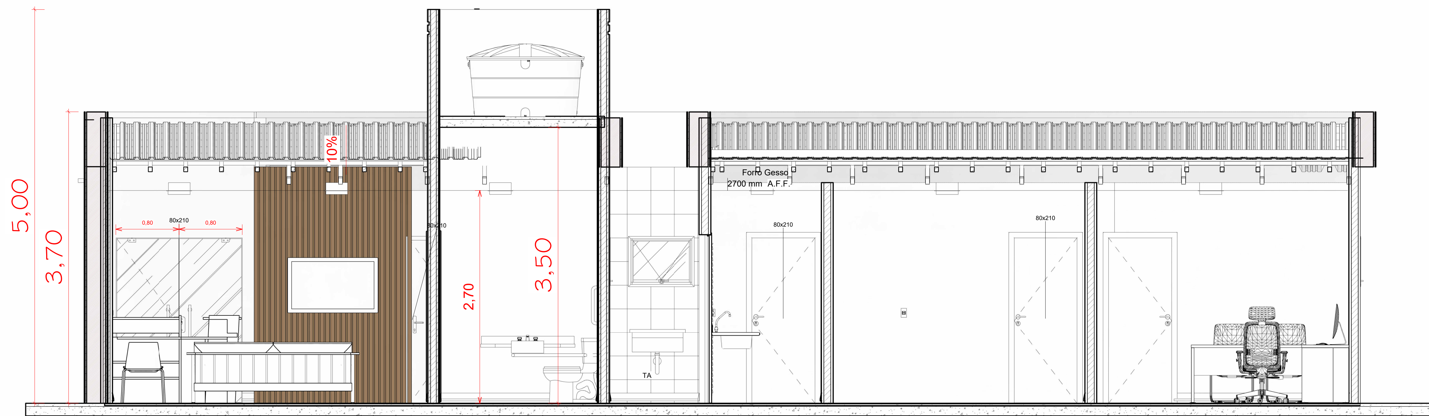
2 CORTE 01 1 : 25
