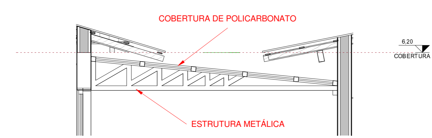
5 CORTE E 1 : 25
