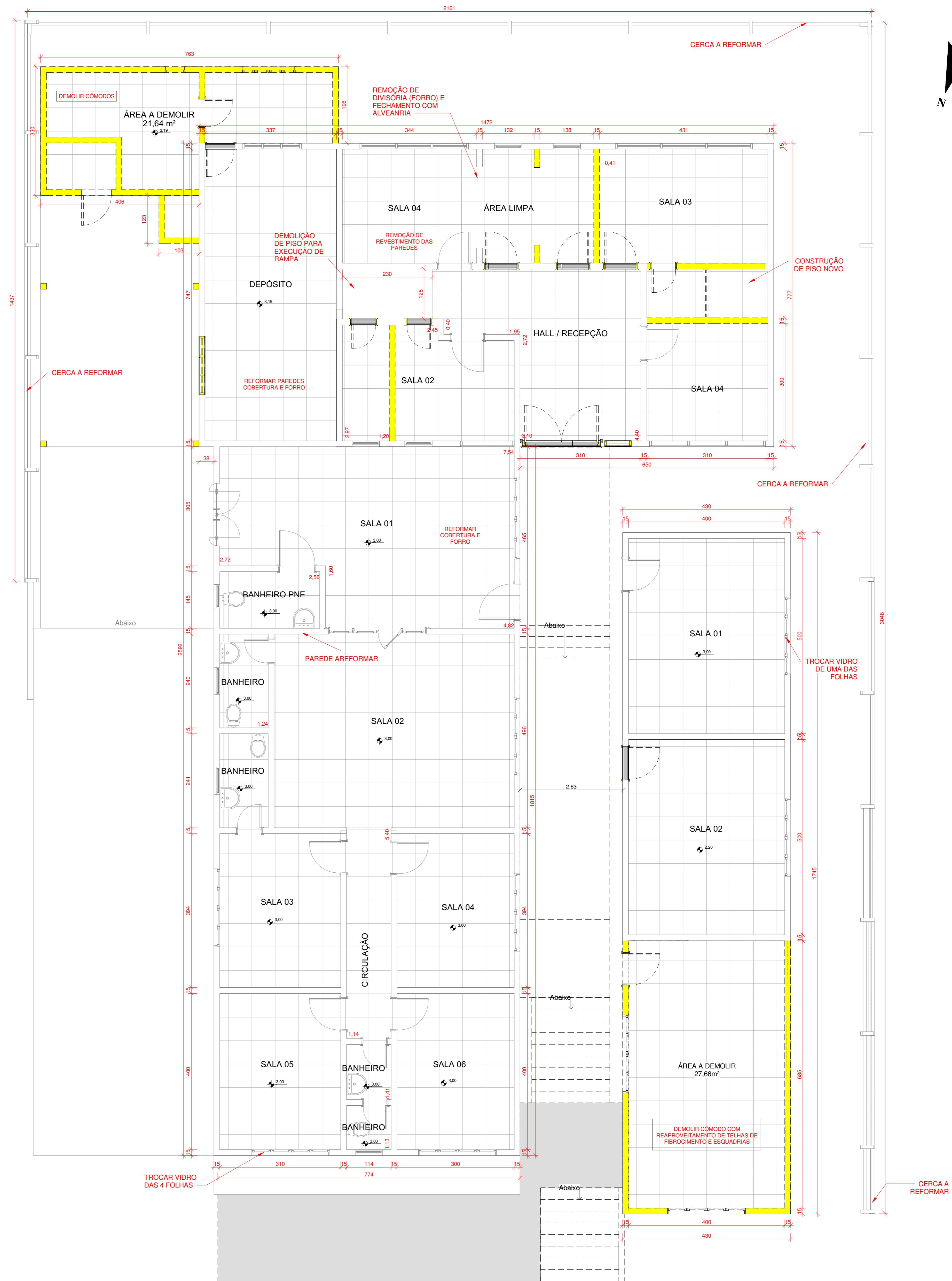
2 PAV 02 - DEMOLIR 1 : 50
