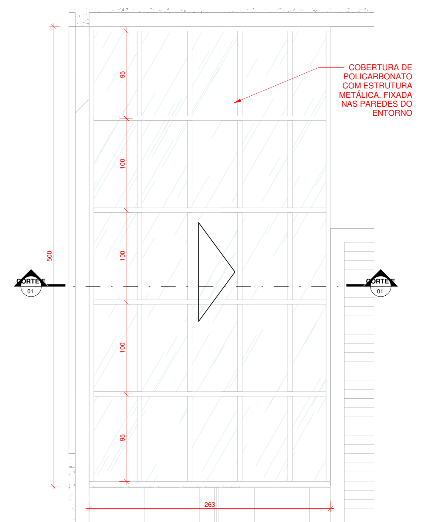
01 DETALHE 01 1 : 25
