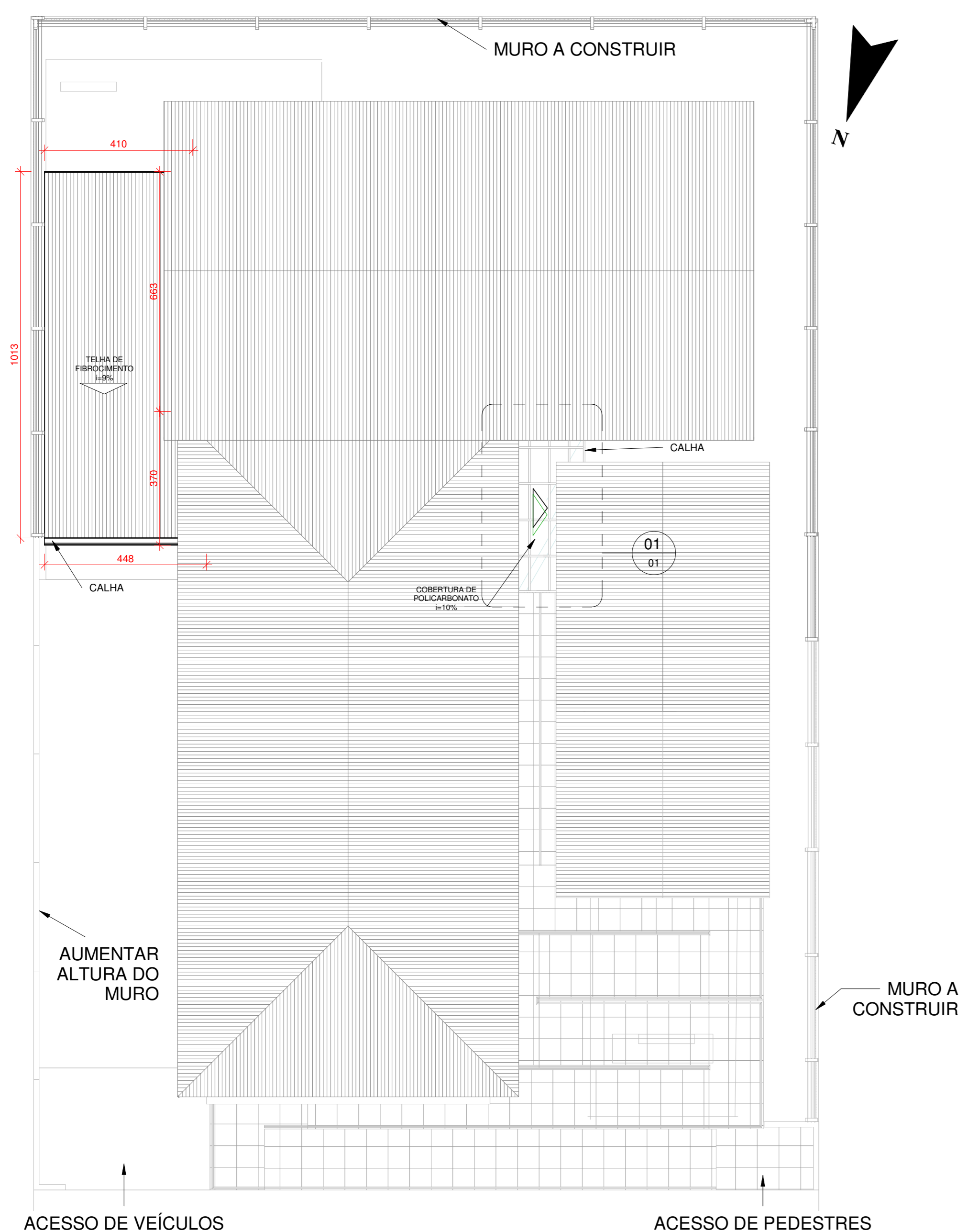
3 COBERTURA 1 : 100
