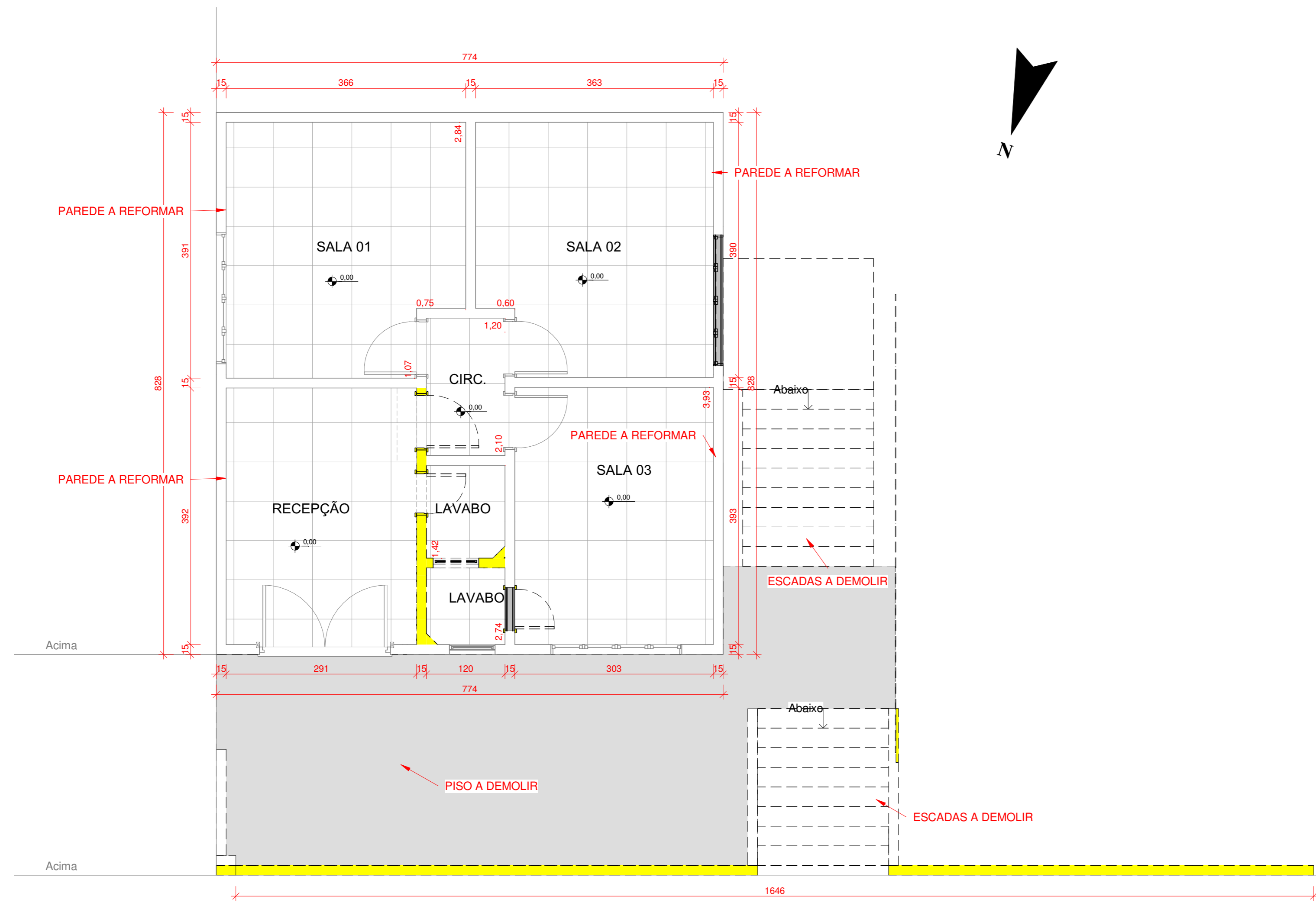
1 PAV 01 - DEMOLIR 1 : 50
