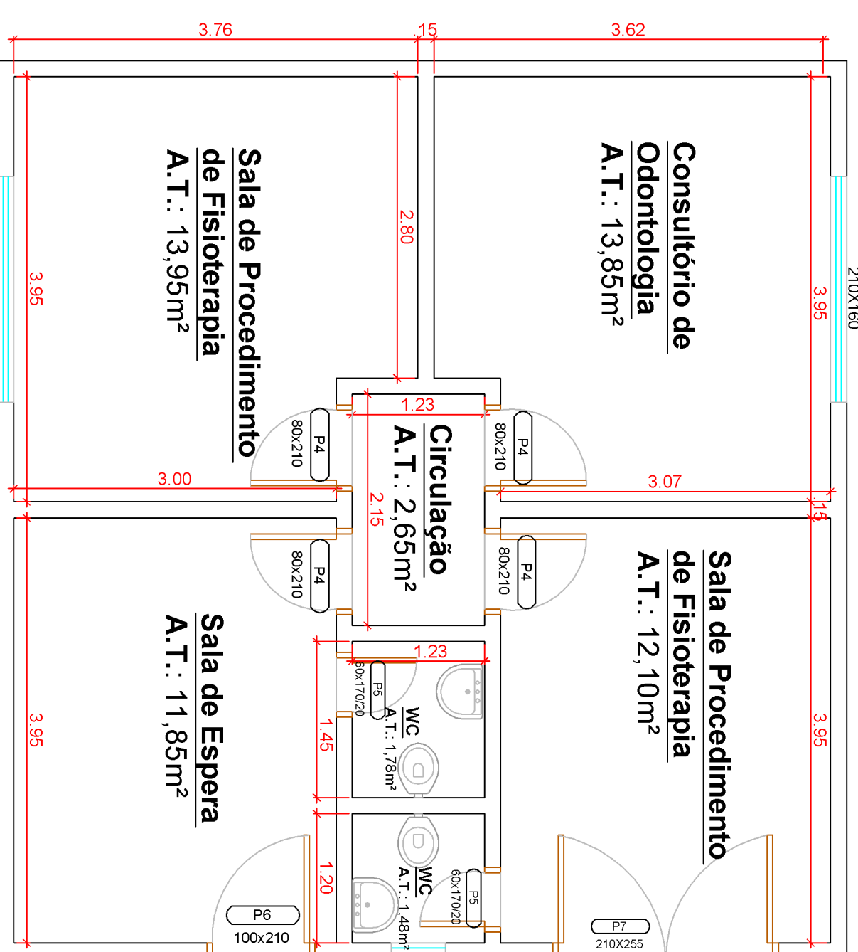
PLANTA BAIXA PISO INFERIOR Esc. 1:50
